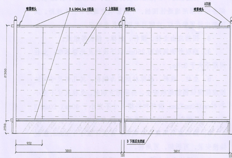
图 1-1 金属组合式围挡立面示意图
