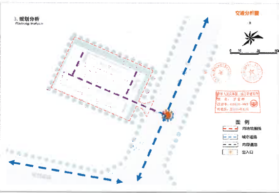
交通分析图
