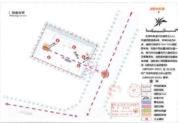
消防分析图
