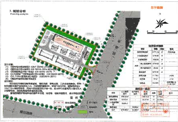
总平面图
