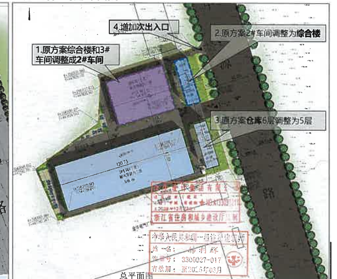
变更后方案总平面图
