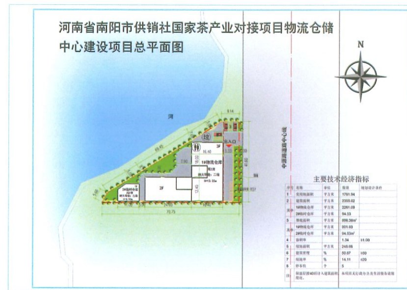
平面分析图
