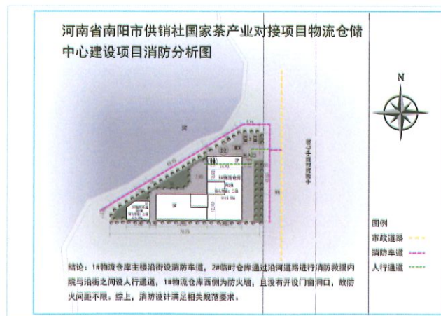
消防分析图
