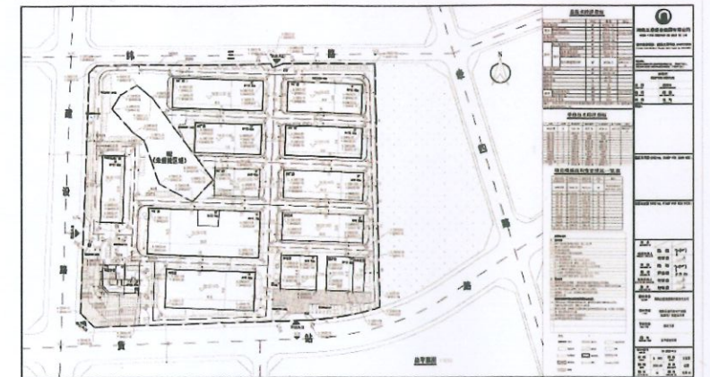
变更后总平图
