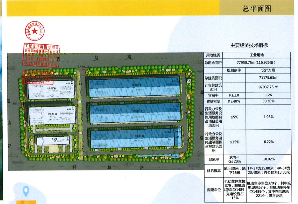
总平面图
