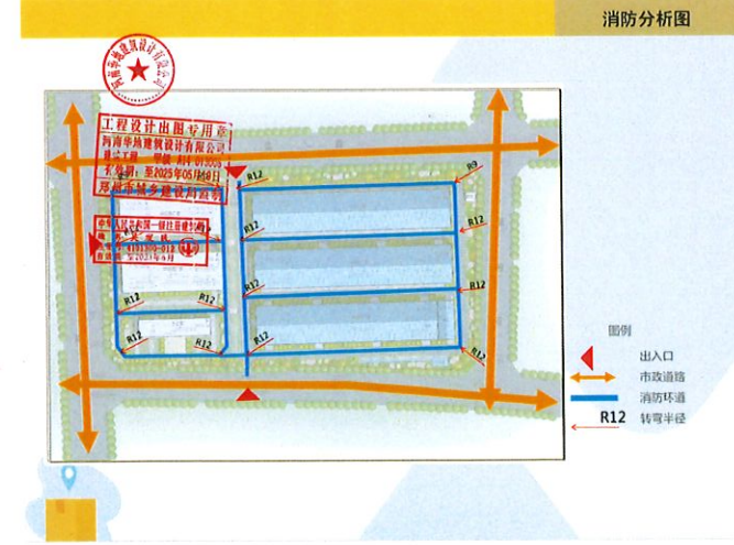
消防分析图
