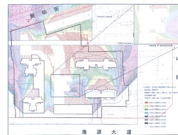
日照分析图
