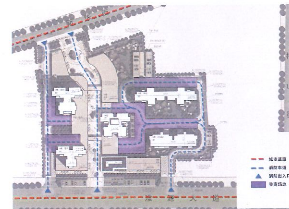
消防分析图
