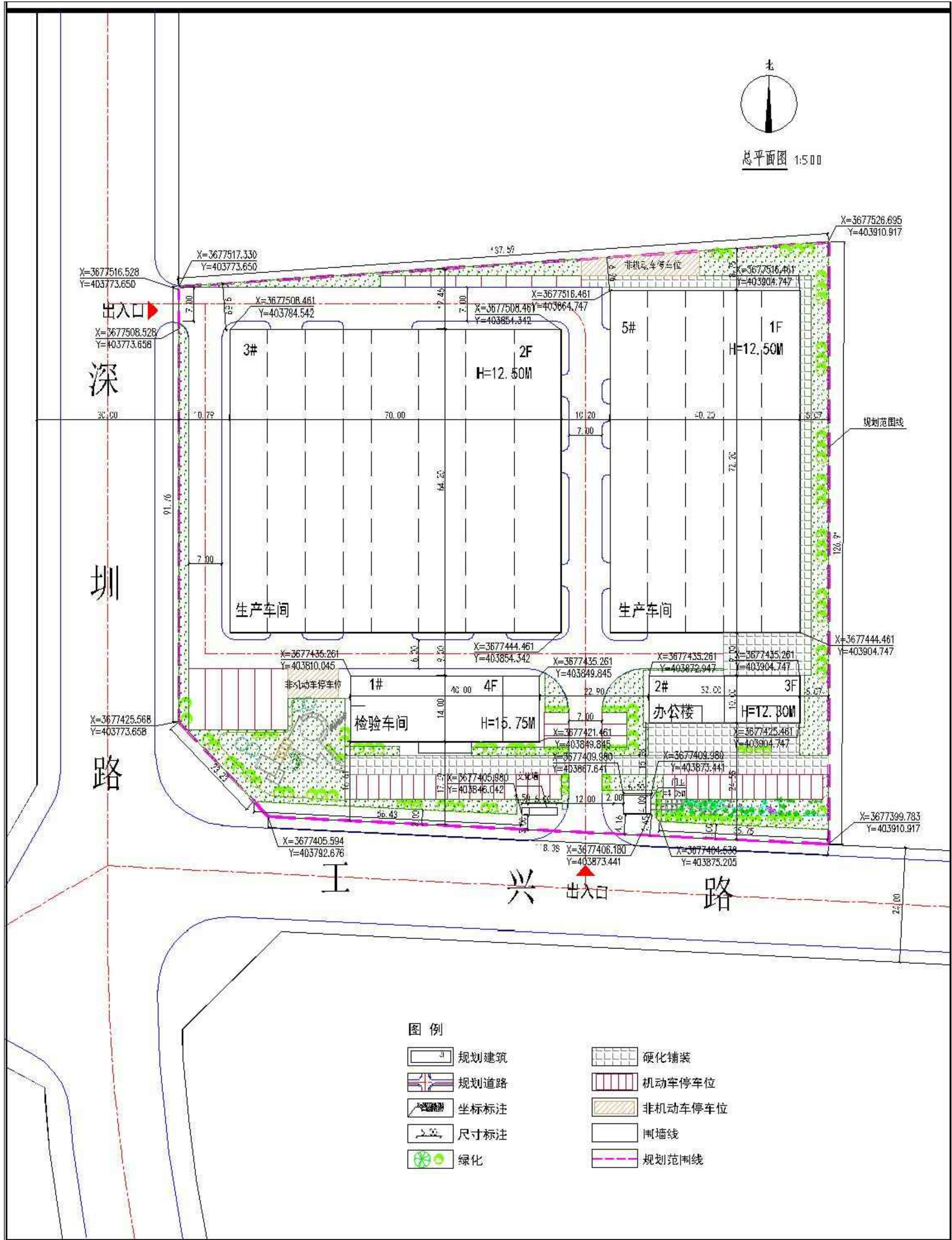
规划平面图
